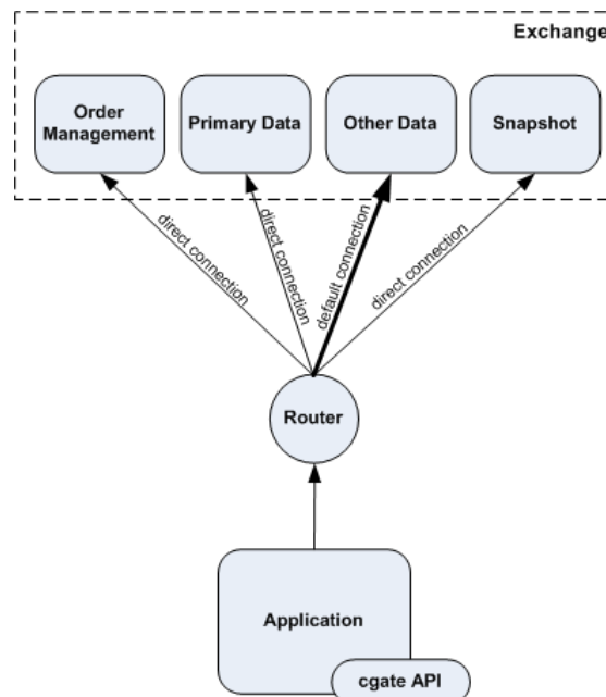
Рис. 18. Схема соединений
