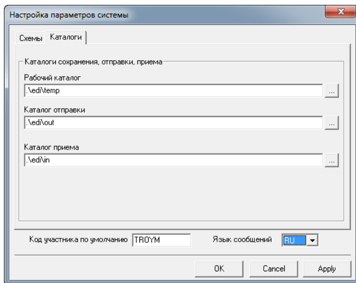
Рис. 4.15. Настройка каталогов
