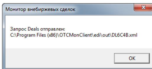
Рис. 4.5. Отправка отчета
